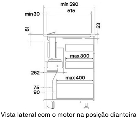
Vista lateral com o motor na posição dianteira
