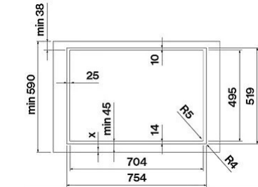
Dimensões do furo
