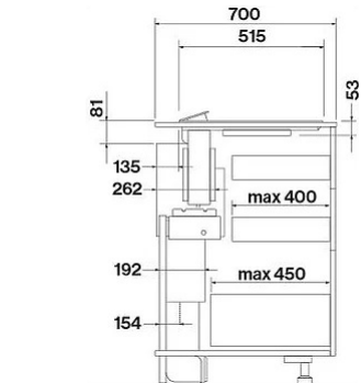
Vista lateral com o motor na posição traseira
