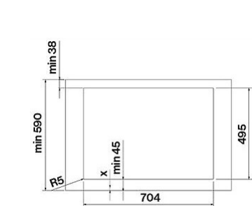
Dimensões do furo
