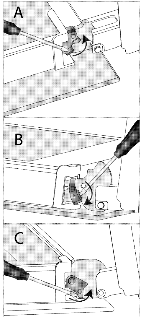
Bloqueio da dobradiça - posição fechada
